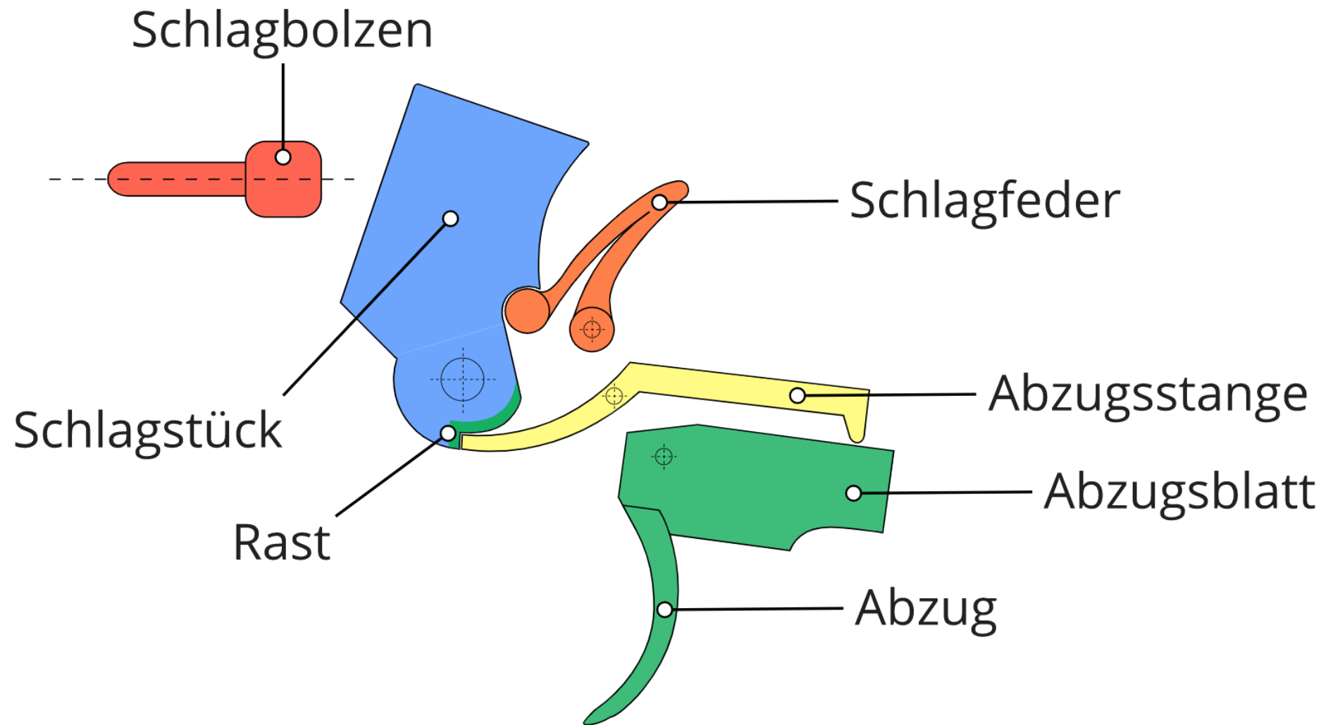
Gespanntes Schloss
