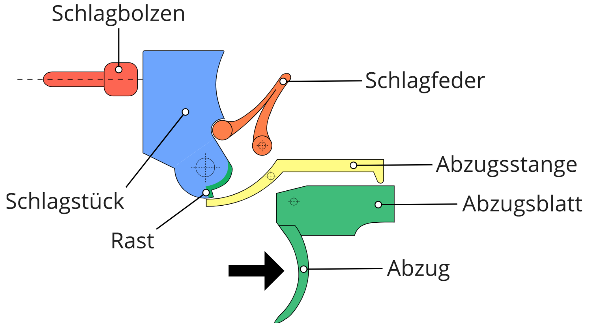
Abgeschlagenes Schloss
